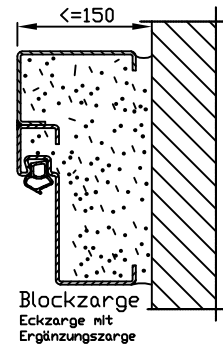
Eckzarge mit Ergänzungszarge Maulweite variabel
